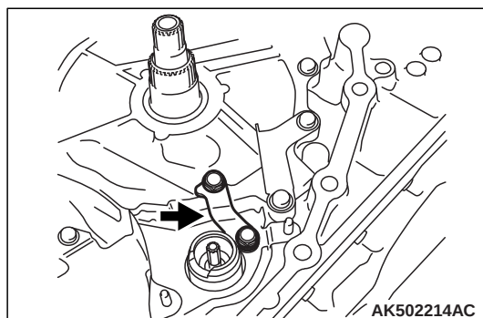
35.拆下支架。
