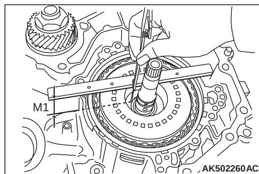
(1) 测量从变速器壳体的机油泵护盖装配表面至前进离合器制动鼓的滚针轴承装配表面的距离 M1。
