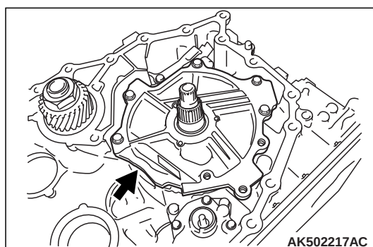
38.从变速器壳体上拆下机油泵护盖。
