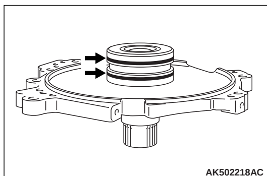
39.从机油泵护盖上拆下密封环。
