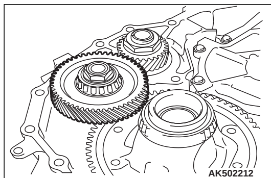
33.从变速器壳体上拆下减速齿轮总成。
