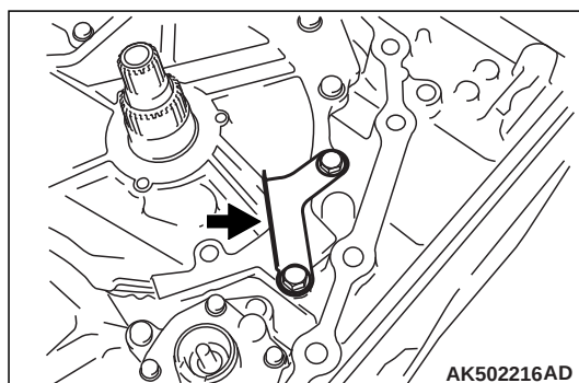
37.拆下机油挡板。
