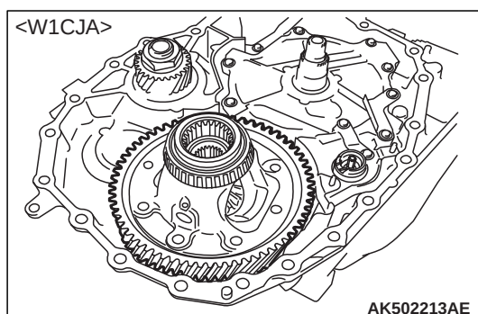
34.从变速器壳体上拆下差速器总成。
