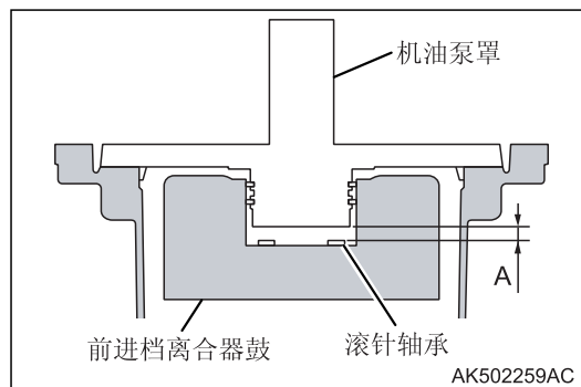
13. 按以下方法测量总端隙 A。
