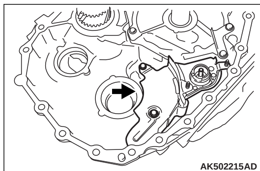
36.拆下机油挡板。
