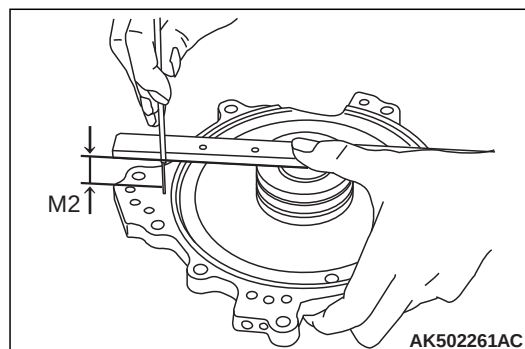
(2) 测量从机油泵护盖的边缘至变速器壳体的装配表面的距离 M2。 (3) 按以下公式计算总端隙。选取符合总端隙标准值的滚针轴承。
